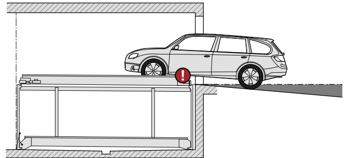
max. 5% gradient
